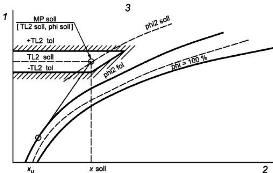
Рисунок 7 - Представление допустимых значений для точки смешения
