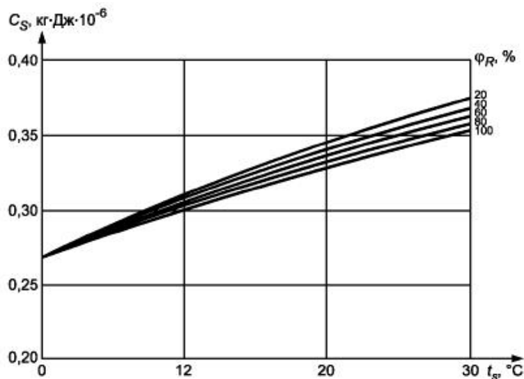
Рисунок С.1 - Удельное потребление воды
