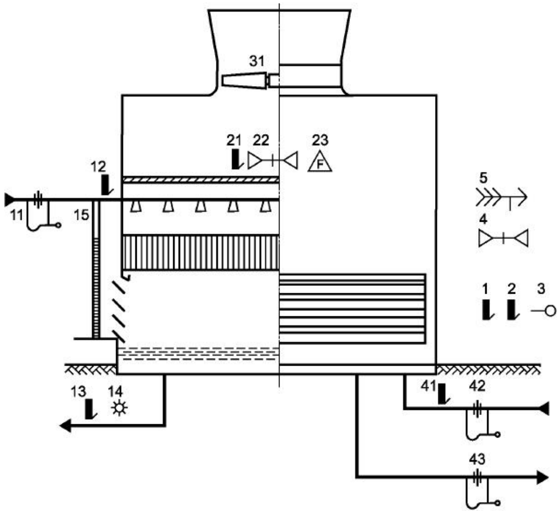
Рисунок 4 - Расположение точек измерений в вентиляторной градирне
