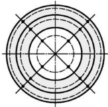
Рисунок 2 - Пример секционирования измеряемой зоны (круговая зона)
