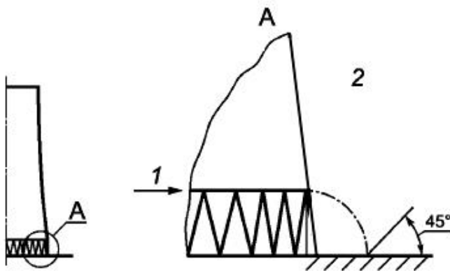
1 - верхний уровень выхода воздуха; 2 - зона без мешающих элементов
