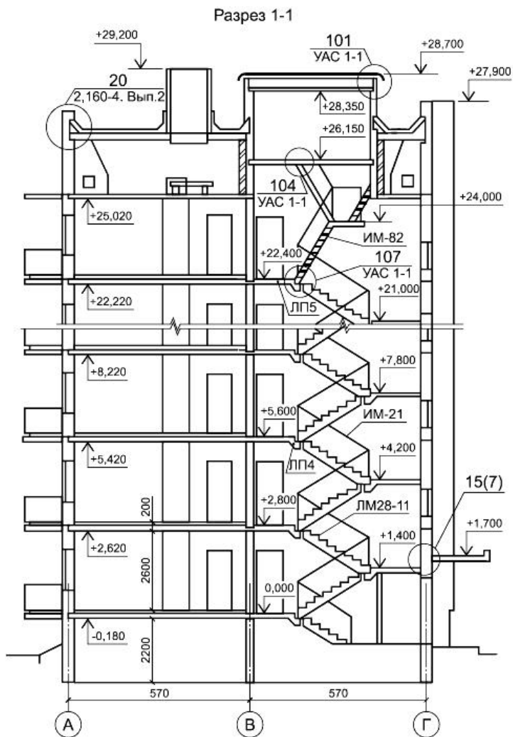
Рисунок Г.3 - Пример выполнения разреза жилого дома
