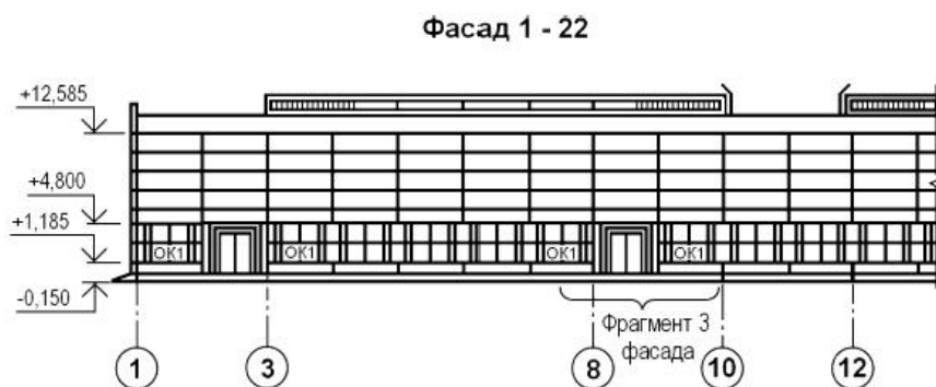
Рисунок Д.1 - Пример выполнения фасада и фрагмента фасада производственного здания
