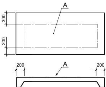
Рисунок 13. Участки поверхности, требующие специальной обработки
